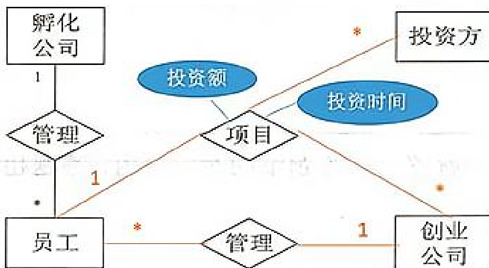
图 2-1 实体联系图
