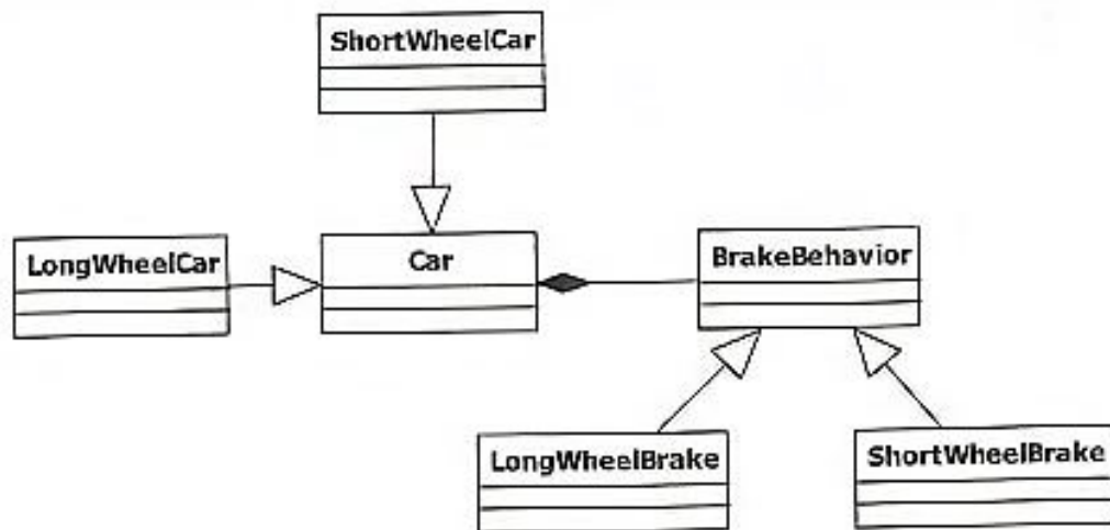
图 5-1 类图
