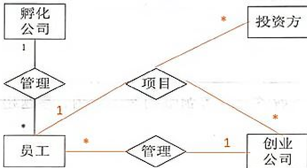
图 2-1 实体联系图
