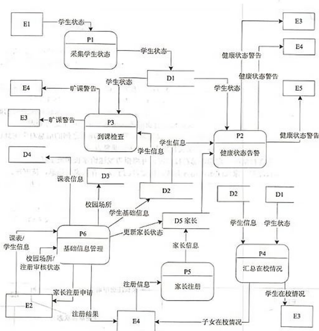
图 1-2 0层数据流图
